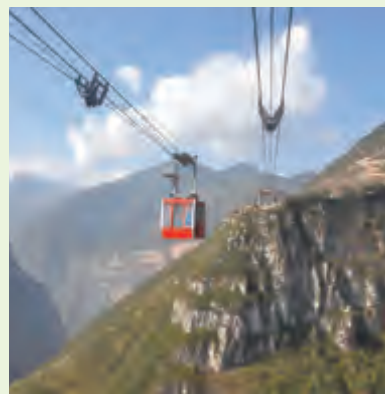
索道线路
